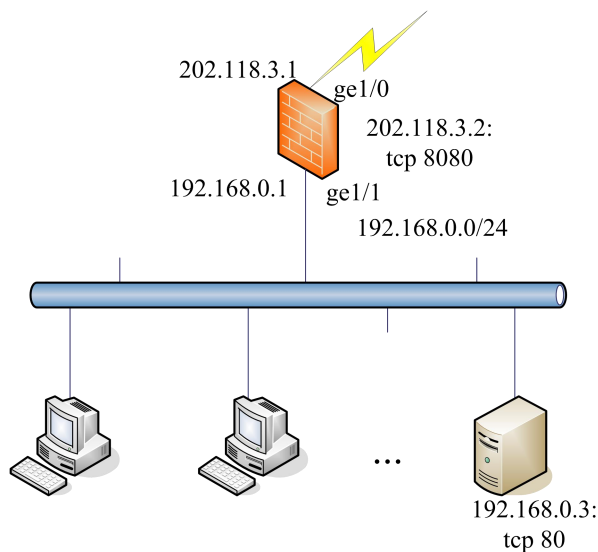
图 15-3 配置 destination NAT 案例组网图
