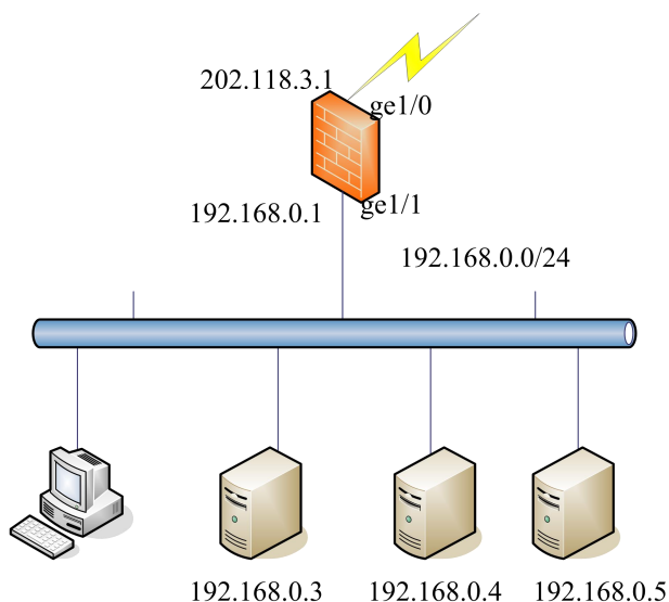
图 15-5 配置 destination NAT 案例组网图 a
