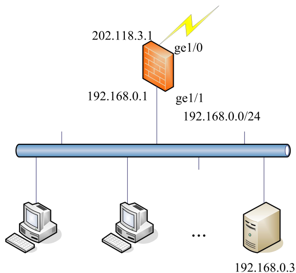
图 15-5 配置 destination NAT 案例组网图 a
