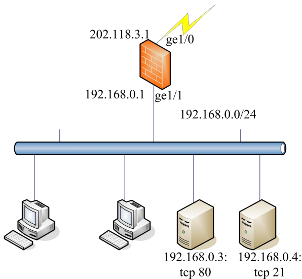
图 15-4 配置 destination NAT 案例组网图 a
